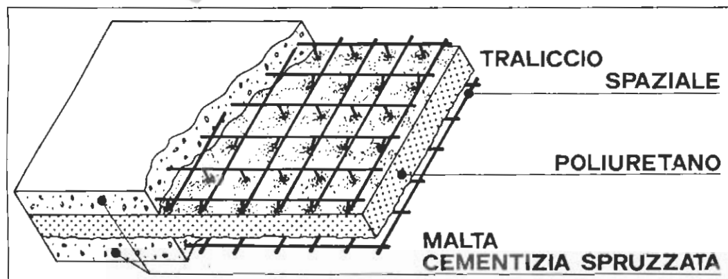
Spaccato di parete portante REIN.
